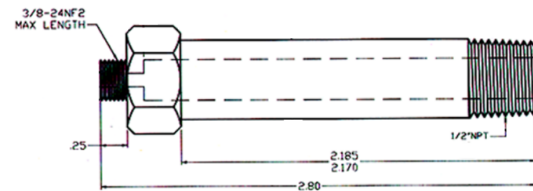
N-78L 1/2" NPT Lagg P/T Plug
