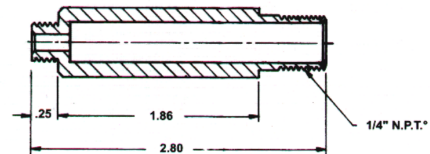
N-76L 1/4" NPT Lagg P/T Plug
